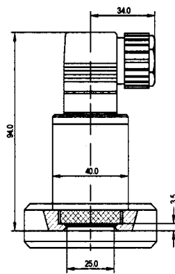
Milchrohr DN 25 Messbereiche : 0/20 mbar bis 0/40 bar
