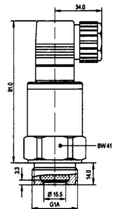
G 1 A Messbereiche : 0/100 mbar bis 0/250 bar
