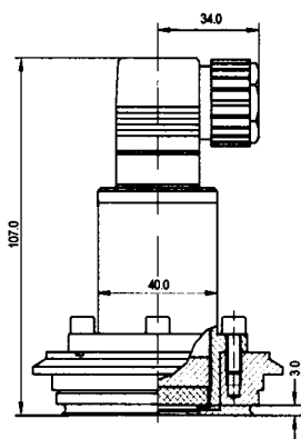
Varivent Messbereiche : 0/20 mbar bis 0/40 bar
