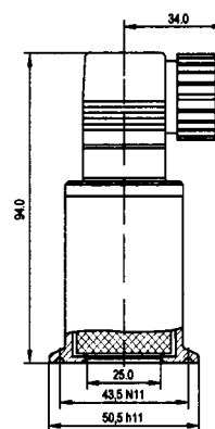
Clamp DN 25 Messbereiche : 0/20 mbar bis 0/40 bar
